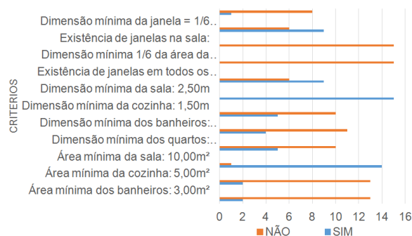
Gráfico 2. Análise técnica.
